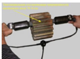
Намагничивание изделий сложной формы отдельными полюсами
